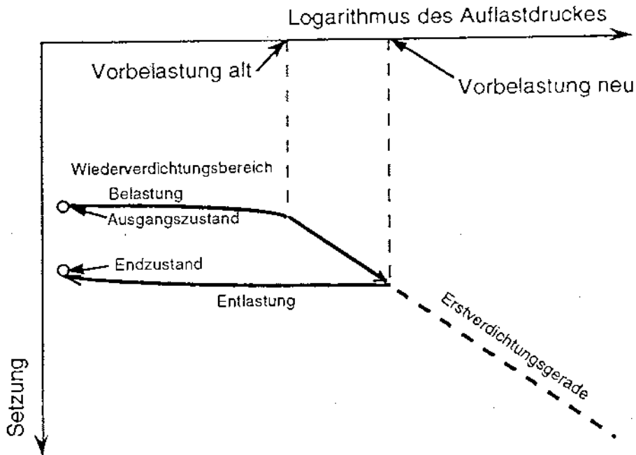
Abb. 1b Nicht reversible (plastische) Verdichtung: Die bestehende Vorbelastung wird überschritten. Der Boden wird dauerhaft verdichtet. Je nach Ausmass kann dies eine mehr oder weniger starke Beeinträchtigung der Bodenfruchtbarkeit zur Folge haben.
