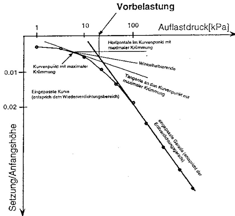
Abb. 3 Bestimmung der Vorbelastung nach Casagrande
