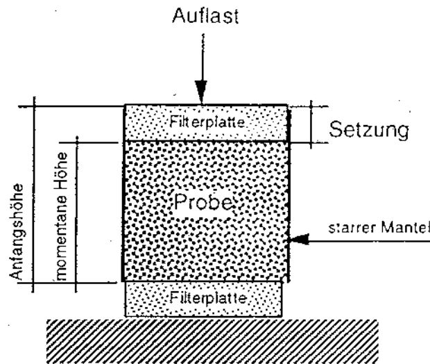
Abb. 2 Schema eines Ödometers
