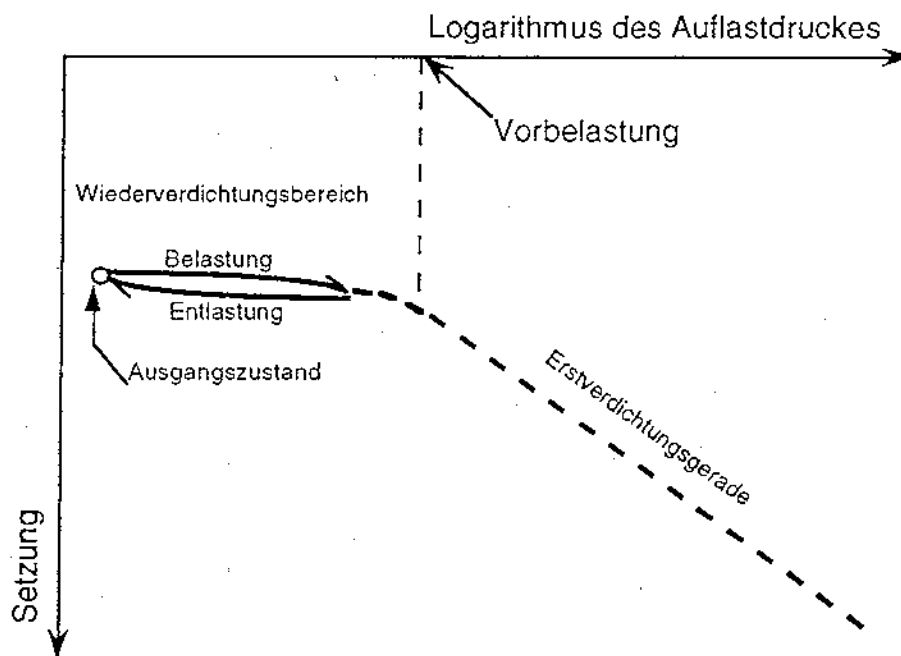
Abb. 1a Reversible (elastische) Verdichtung: Die Vorbelastung wird nicht überschritten. Der Boden wird nur vorübergehend verdichtet, d.h. solange die Belastung anhält.
